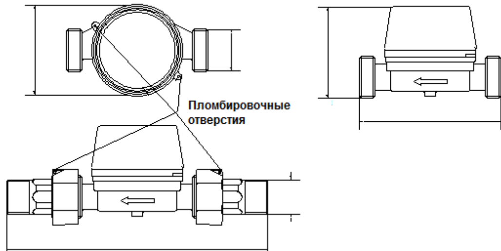
Рисунок 1. Счетчики воды
